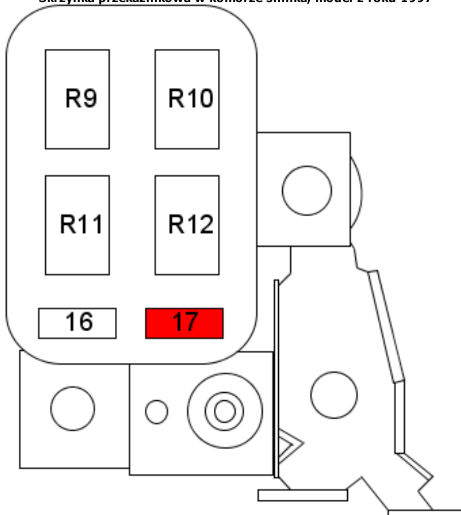
Skrzynka przełącznikowa w komorze silnika, model z roku 1997
