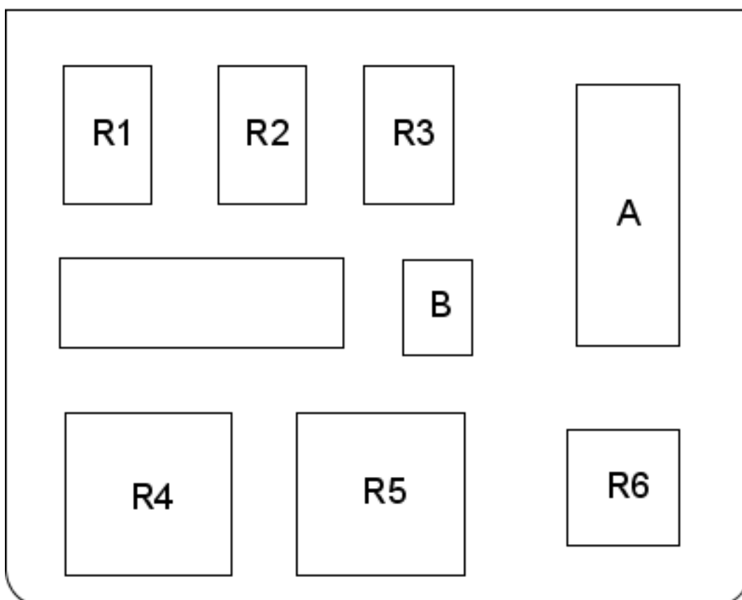
Skrzynka przełącznikowa w przedziale dla pasażerów, model z roku 1992 - 1995
